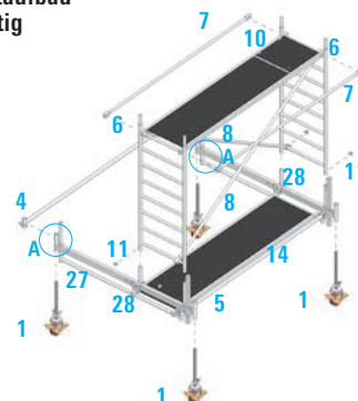
Gerüstaufbau einseitig
