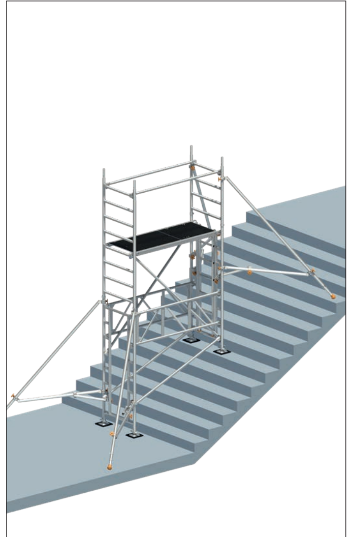
16. Anbau der Gerüststützen (s. S. 20, Kapitel 7. Gerüststützen-Anbau).
