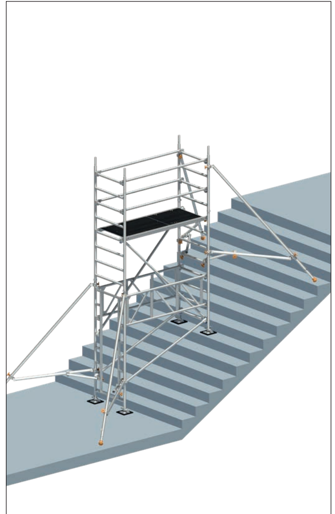
16. Montage der Geländer auf 50 cm Höhe.
