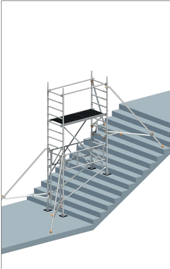
15. Anbau der Gerüststützen (s. S. 20, Kapitel 7. Gerüststützen-Anbau).
